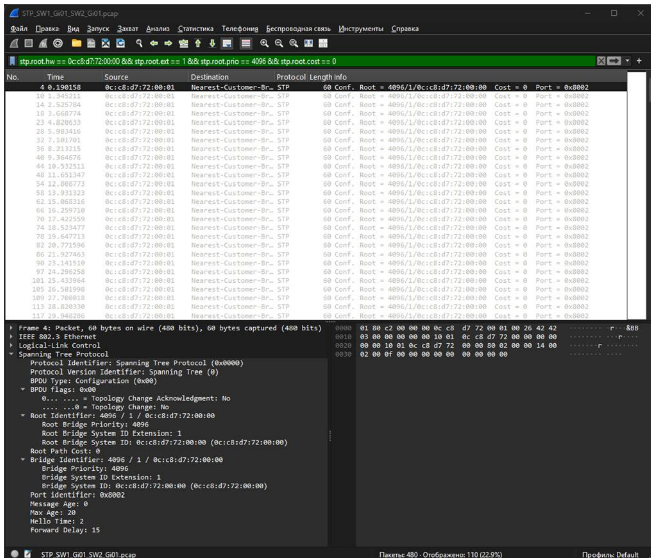
Рисунок 4 — STP Hello BPDU на линке Layer2Switch-1 Gi0/1 — Layer2Switch-2 Gi0/1
