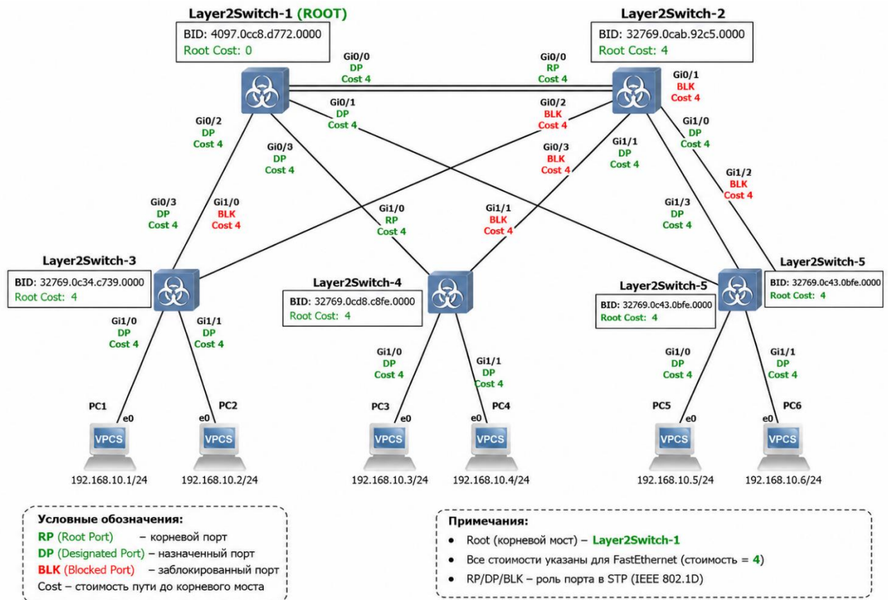
Рисунок 3.1 — Топология STP с BID коммутаторов, ролями портов и стоимостями маршрутов
