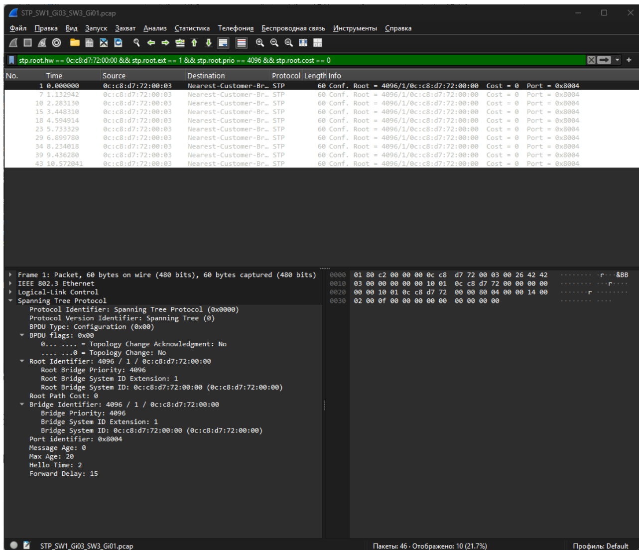
Рисунок 7 — STP Hello BPDU на линке Layer2Switch-1 Gi0/3 — Layer2Switch-3 Gi0/1
