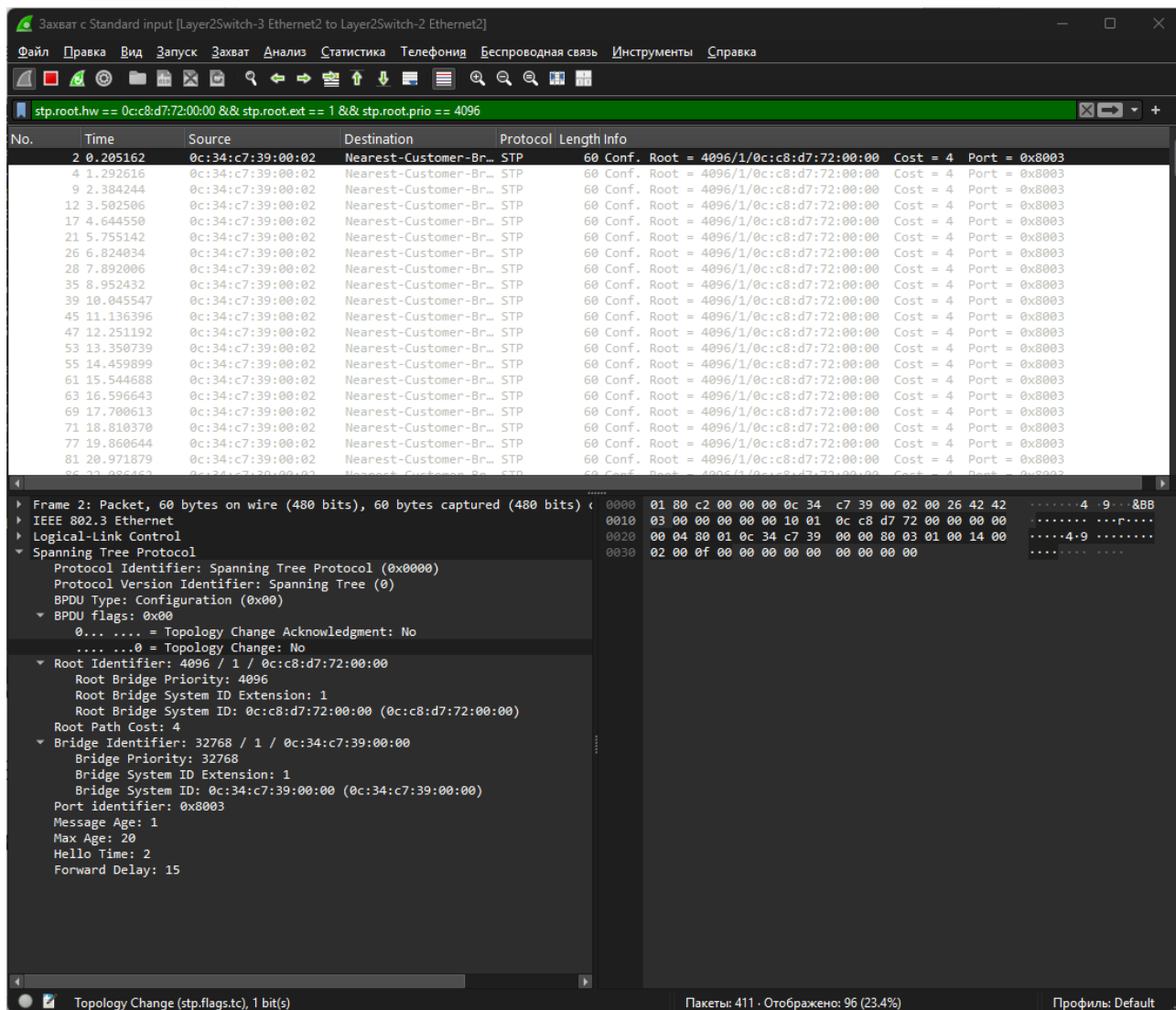
Рисунок 12 — STP Hello BPDU на линке Layer2Switch-2 Gi0/2 — Layer2Switch-3 Gi0/2
