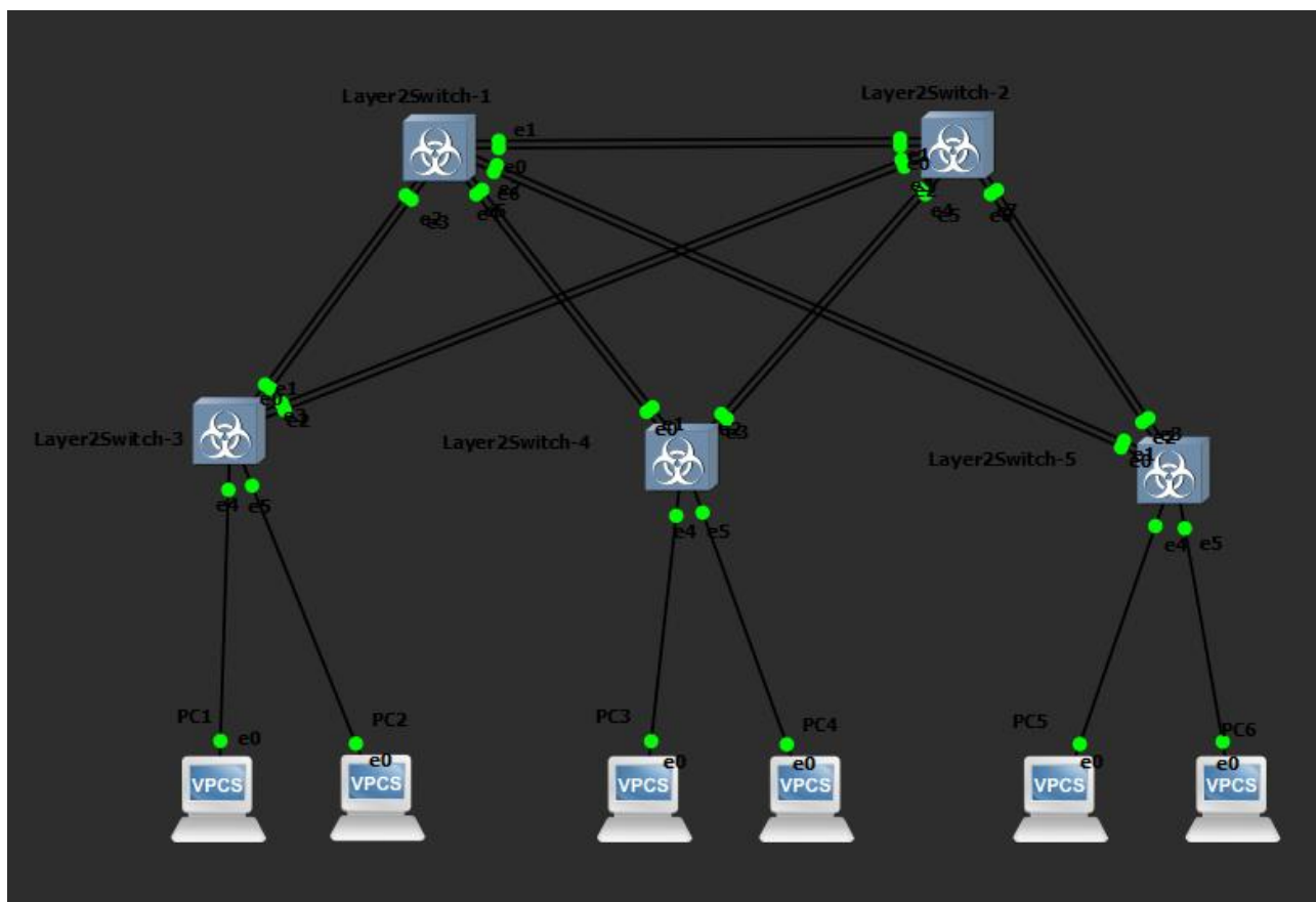
Рисунок 1 — Топология сети для исследования протокола STP
