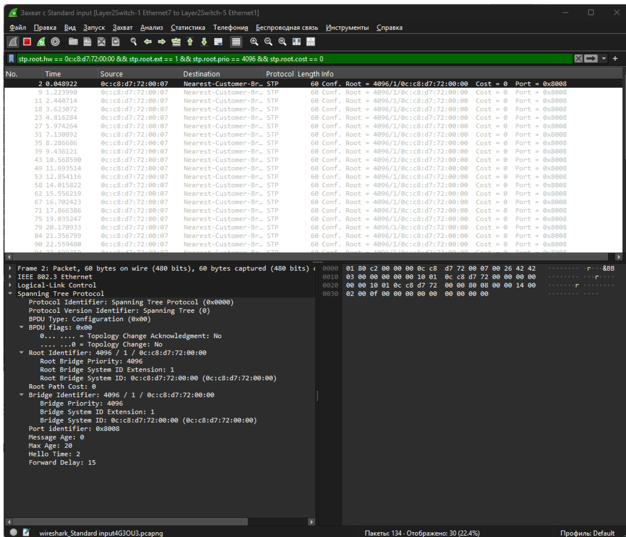
Рисунок 11 — STP Hello BPD на линке Layer2Switch-1 Gi1/3 — Layer2Switch-5 Gi0/1
