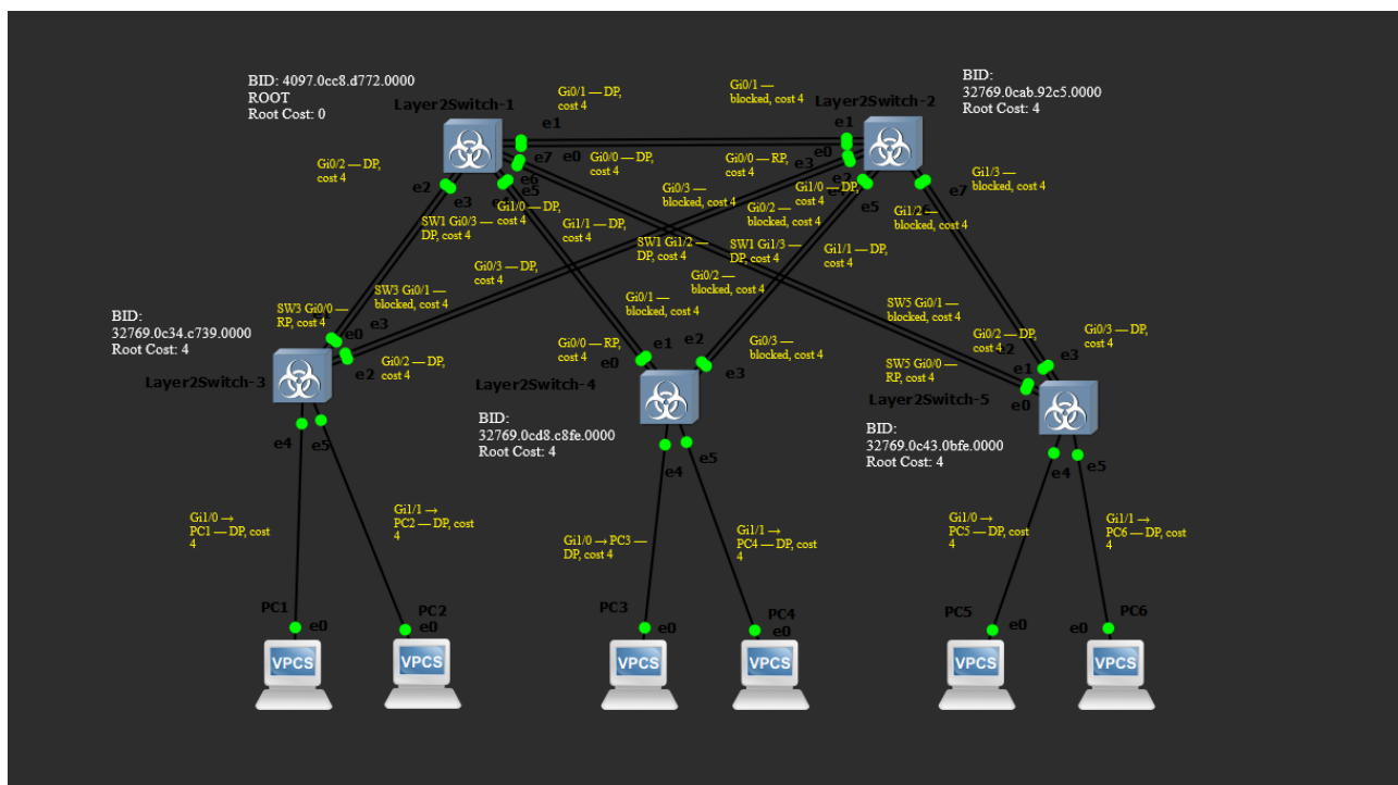
Рисунок 3 — Топология STP с BID коммутаторов, ролями портов и стоимостями маршрутов
