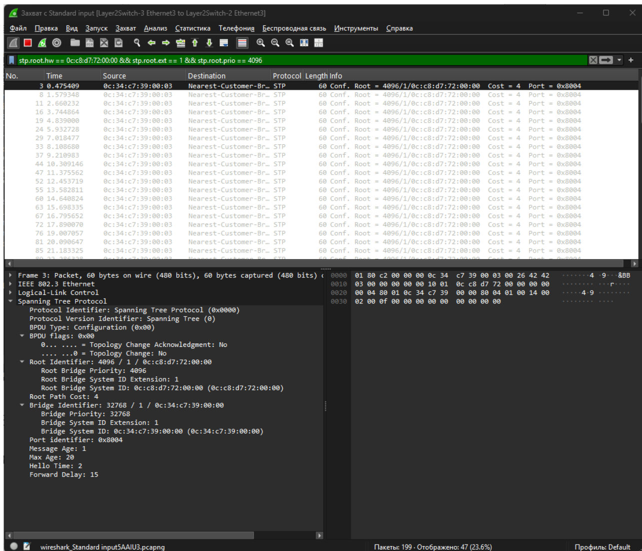
Рисунок 13 — STP Hello BPDU на линке Layer2Switch-2 Gi0/3 — Layer2Switch-3 Gi0/3
