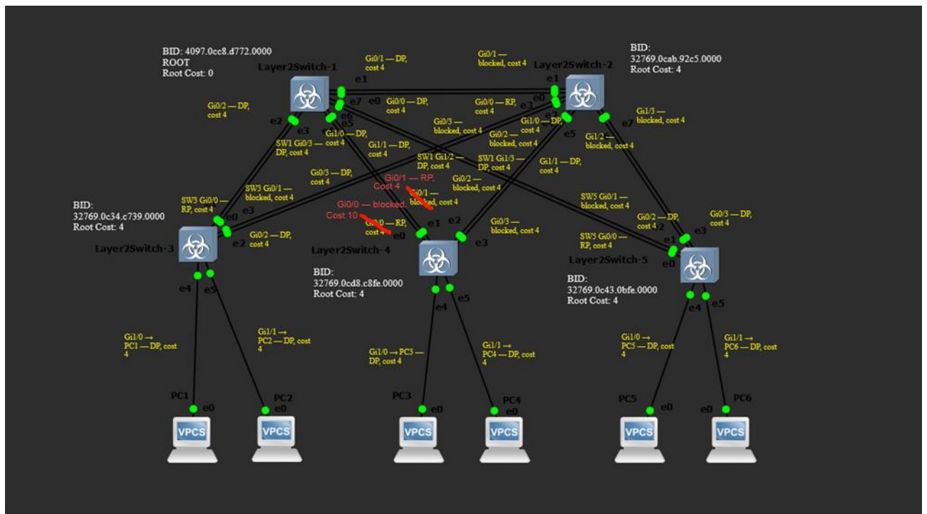
Рисунок 18 — Топология STP после изменения стоимости Root Port
