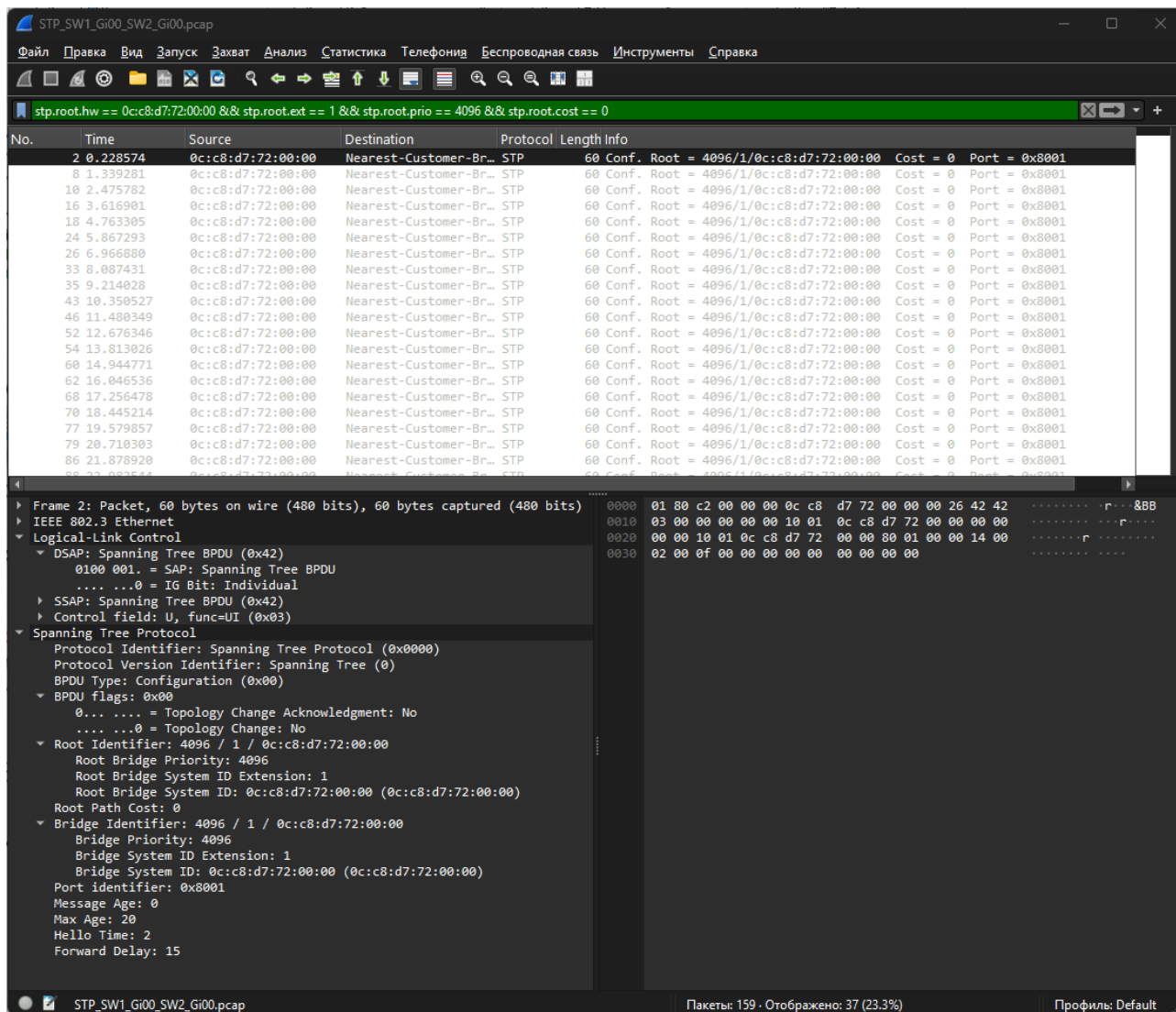
Рисунок 5 — STP Hello BPDU на линке Layer2Switch-1 Gi0/0 — Layer2Switch-2 Gi0/0
