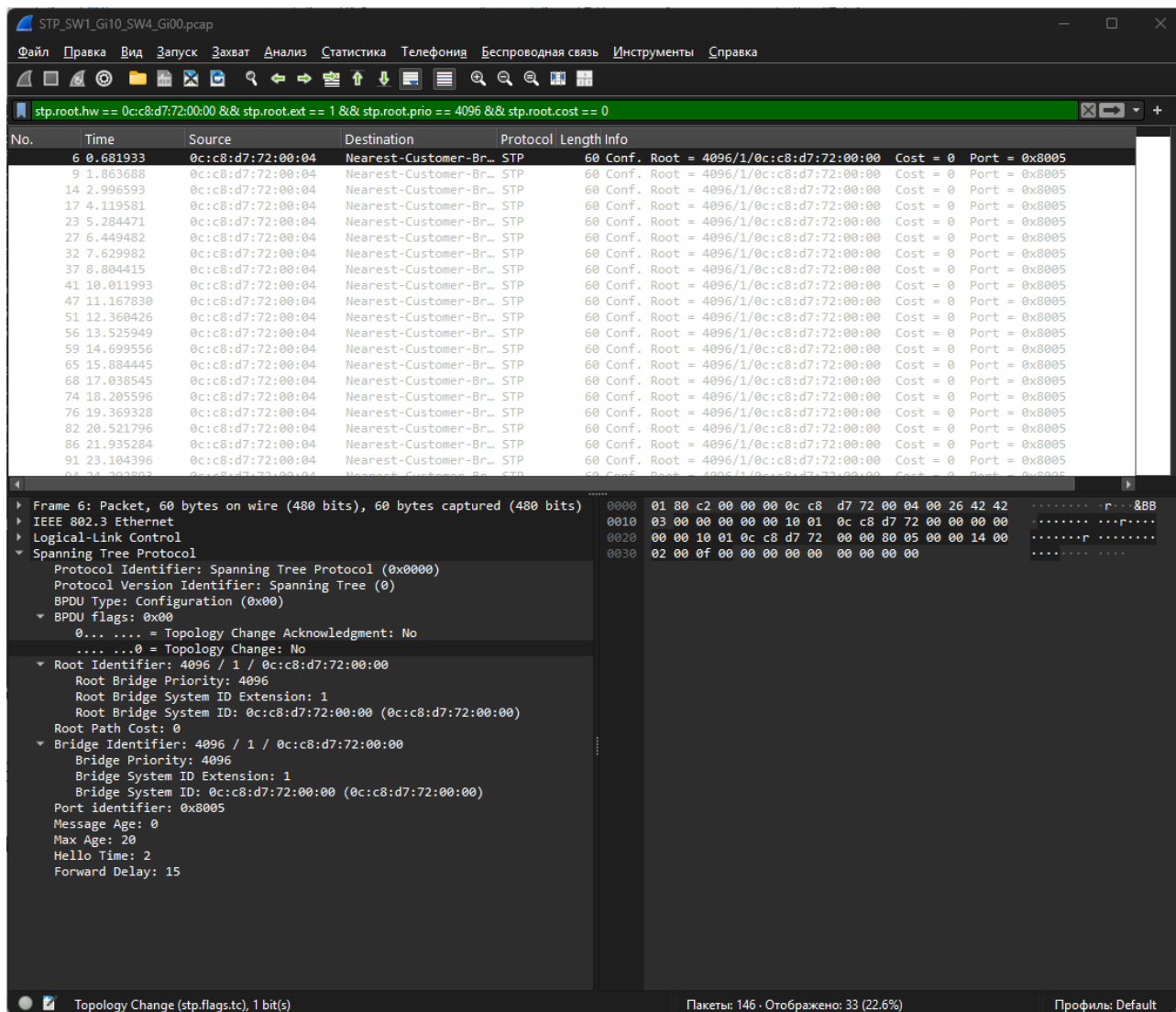
Рисунок 8 — STP Hello BPDU на линке Layer2Switch-1 Gi1/0 — Layer2Switch-4 Gi0/0
