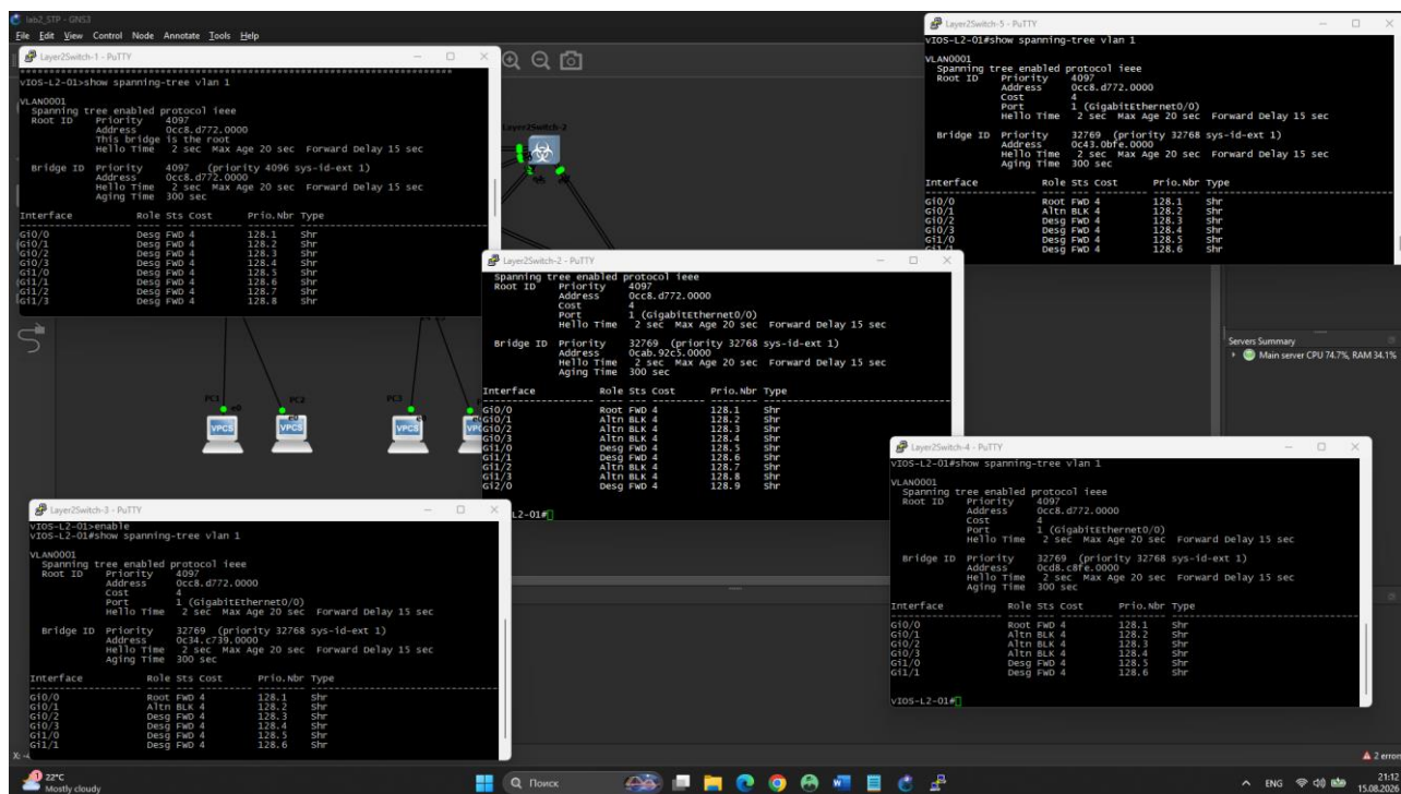
Рисунок 2 — Результаты проверки состояния STP на коммутаторах сети
