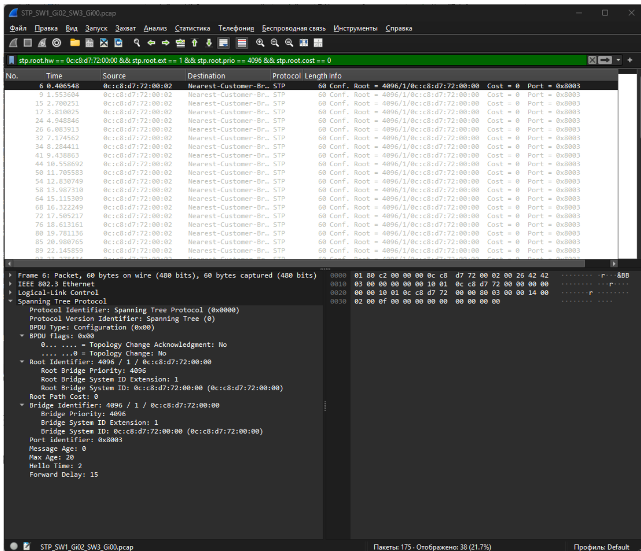
Рисунок 6 — STP Hello BPDU на линке Layer2Switch-1 Gi0/2 — Layer2Switch-3 Gi0/0
