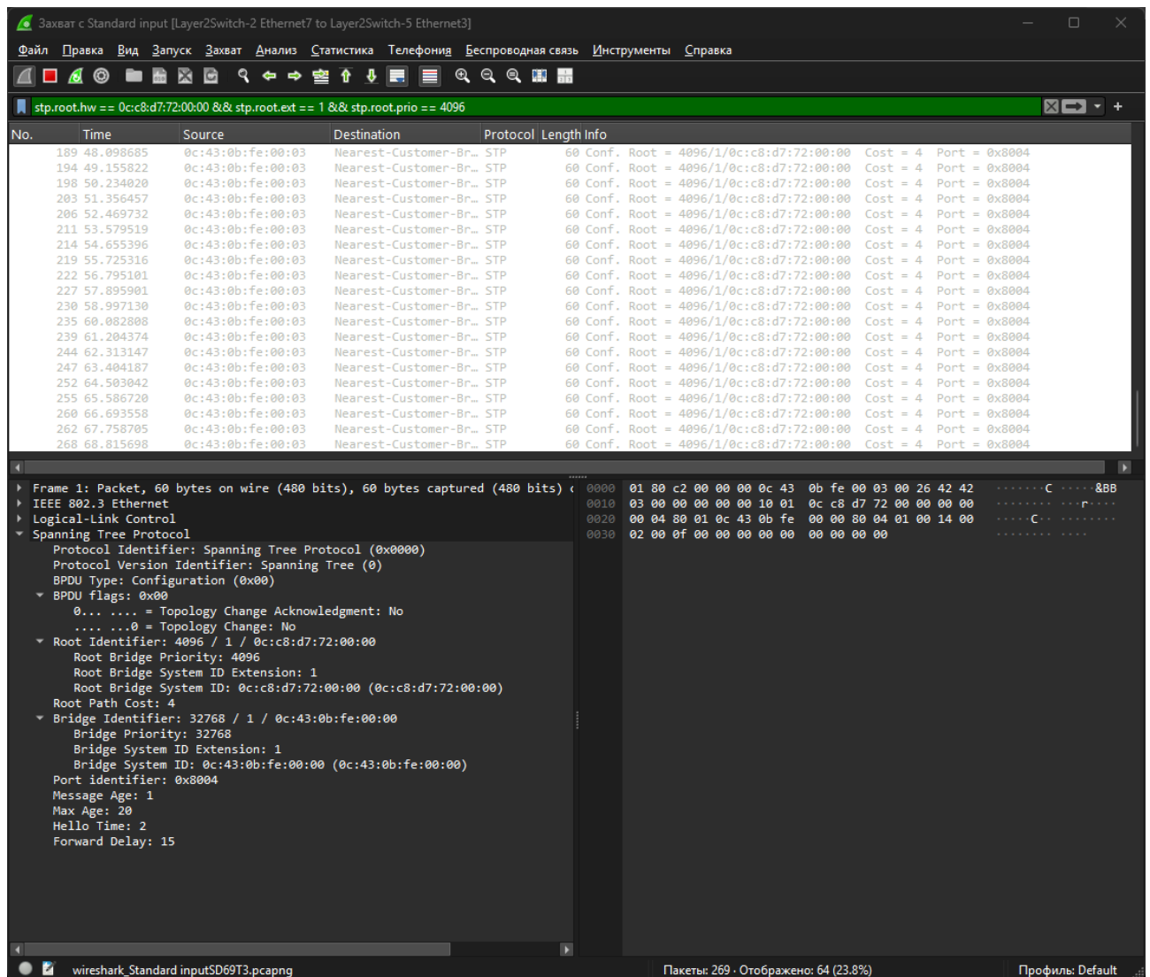
Рисунок 17 — STP Hello BPDU на линке Layer2Switch-2 Gi1/3 — Layer2Switch-5 Gi0/3
